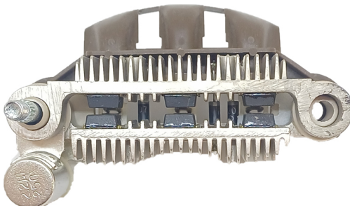
FA-MI-1447 Placa Mitsubishi A860T17570; A860T19970 Mazda CON DIODO AUXILIAR
