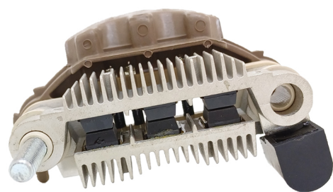
FA-MI-1415 Placa Mitsubishi A860T20570, A860X20599. Nissan CON DIODO AUXILIAR
