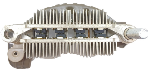
FA-MI-1433 Placa Mitsubishi A860X58170 Nissan, Mitsubishi CON DIODO AUXILIAR
