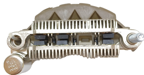
FA-MI-1454 Placa Mitsubishi A860T31370, 34070 Ford; Mazda; Mercury CON DIODO AUXILIAR
