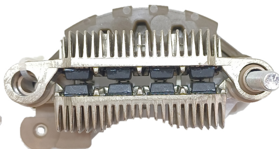
FA-MI-1480 Placa Mitsubishi A860X83370 Honda CON DIODO AUXILIAR
