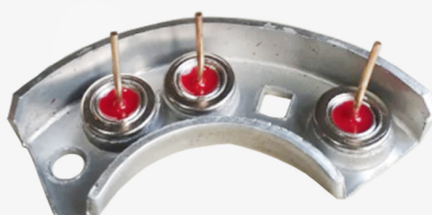
FA-090 POSITIVA Placa tipo Argelite 28-38-42 amp Peugeot-Citroen Renault
