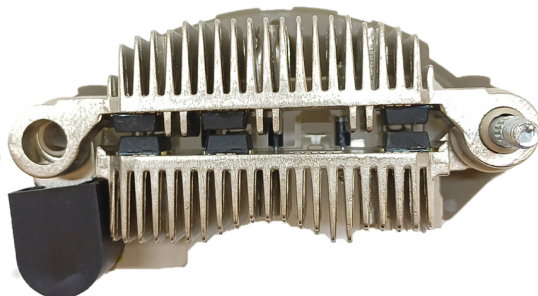
FA-MI-1459 Placa Mitsubishi A860T37670, 39170 Ford; Mazda; Mitsubishi CON DIODO AUXILIAR
