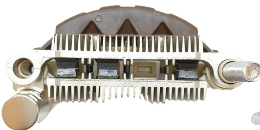
FA-MI-1426 Placa Mitsubishi A860T32170. Ford, Mazda CON DIODO AUXILIAR
