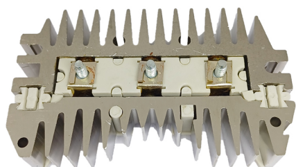
FA-DE-1104 Placa Delco 1852744, 1875812 Alternadores Delco serie 27SI, tipos 200, y serie 30SI. Positivo a masa. IR/EF. CON DIODO AUXILIAR
