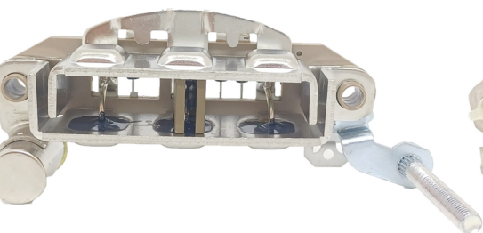
FA-MI-1404 Placa Mitsubishi A860T08270 Mitsubishi, Dodge. CON DIODO AUXILIAR
