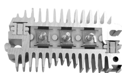
FA-DE-1121 Placa Delco 1852209; 1971987; D3915 GM varios GMC Chevett Å '80, Å '81 CON DIODO AUXILIAR
