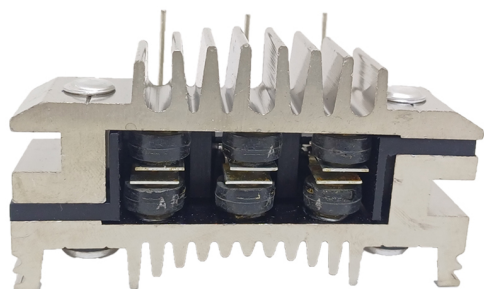
FA-V-1625 Placa Valeo NB928; NB931 Citroën, Peugeot, Renault CON DIODO AUXILIAR
