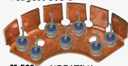
FA-580 NEGATIVA Placa tipo Nashville 100 amp Mercedes Benz Cobre con diodos Soldados
