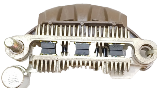
FA-MI-1414 Placa Mitsubishi A860T20070, A860T23570, A860X20099 Mazda, Nissan. CON DIODO AUXILIAR
