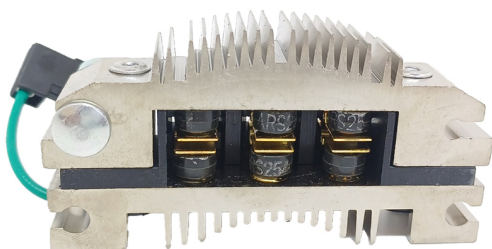
FA-MM-1314 Placa Marelli 63621501 Fiat; Renault CON DIODO AUXILIAR
