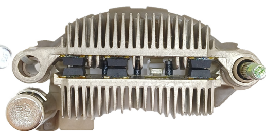
FA-MI-1472 Placa Mitsubishi A860X47770 Mazda CON DIODO AUXILIAR
