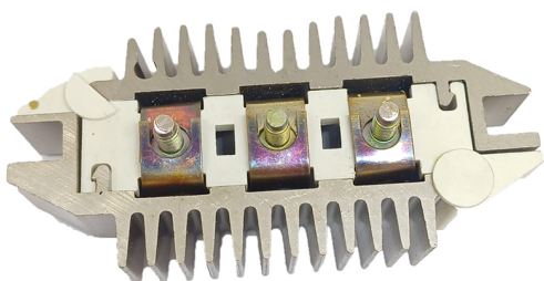
FA-DE-1125 Placa Delco 347813; 3493721; 3493714; 6065301 Chevrolet; Opel CON DIODO AUXILIAR
