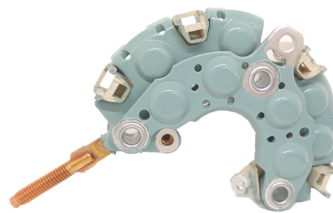
FA-N-1526 Placa Nippondenso 021580-5300 Acura, Isuzu, Toyota John Deere, Suzuki. CON DIODO AUXILIAR
