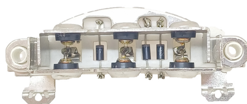
FA-MI-1400 Placa Mitsubishi A860T03970, A860T05170. Mazda, Mitsubishi. CON DIODO AUXILIAR
