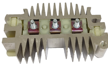
FA-DE-1105 Placa Delco 1975313, D3919 Alternadores Delco serie 15SI, 70A Negativo a masa. IR/EF CON DIODO AUXILIAR
