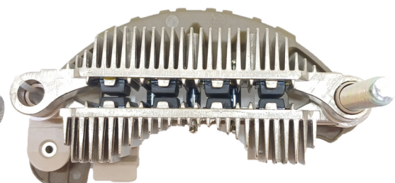
FA-MI-1478 Placa Mitsubishi A4TR5188 Renault Clio, Scania CON DIODO AUXILIAR
