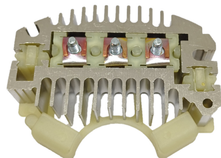
FA-DE-1106 Placa Delco 1984454, D3924 Alternadores Delco serie 12SI, 56-78A IR/EF. CON DIODO AUXILIAR
