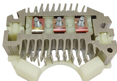
FA-DE-1108 Placa Delco 1987061, D3986 Alternadores Delco serie 12SI, 94A IR/EF. CON DIODO AUXILIAR
