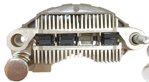
FA-MI-1462 Placa Mitsubishi A860T37870 Honda Civic CON DIODO AUXILIAR
