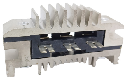
FA-V-1609 Placa Valeo NC 015 Citroen, Volvo, Peugeot Renault CON DIODO AUXILIAR
