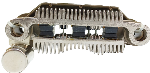
FA-MI-1417 Placa Mitsubishi A860T22670 Mitsubishi CON DIODO AUXILIAR
