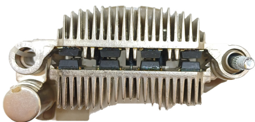
FA-MI-1428 Placa Mitsubishi A860T38970. Mazda CON DIODO AUXILIAR
