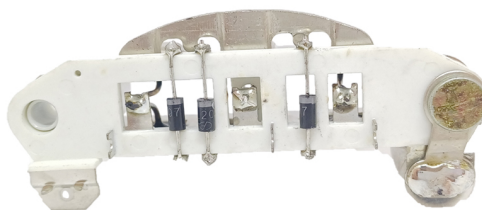
FA-MI-1438 Placa Mitsubishi A860T10770 Mazda CON DIODO AUXILIAR
