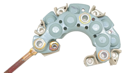
FA-N-1511 Placa Nippondenso 021580-3080 Ford; Daihatsu; Komatsu CON DIODO AUXILIAR
