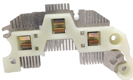
FA-DE-1120 Placa Delco 10475800 Chevy Camaro, Lumina, Chevrolet Omega, Vectra CON DIODO AUXILIAR
