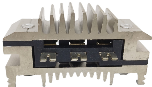
FA-V-1610 Placa Valeo NC016 Renault - Clio - Peugeot. CON DIODO AUXILIAR
