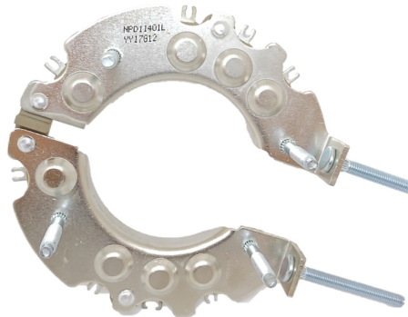
FA-N-1531 Placa Nippondenso 0215802300 Toyota Hilux CON DIODO AUXILIAR
