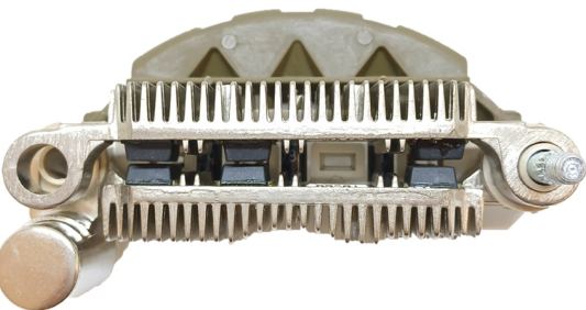
FA-MI-1464 Placa Mitsubishi A860T38270 Ford Escort; Mazda CON DIODO AUXILIAR
