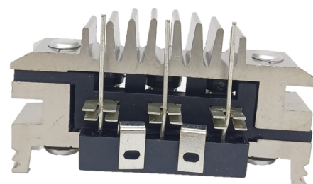
FA-V-1606 Placa Valeo NB 928; NB 931. Citroen, Peugeot, Renault CON DIODO AUXILIAR
