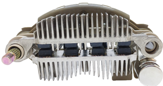
FA-MI-1461 Placa Mitsubishi A2T35791 Mitsubishi; Nissan CON DIODO AUXILIAR
