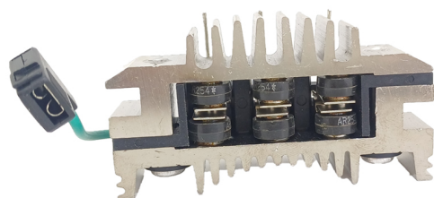
FA-MM-1308 Placa Marelli 64826011/22/40 Fiat 147 y Regatta CON DIODO AUXILIAR
