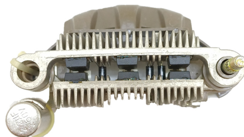
FA-MI-1484 Placa Mitsubishi A860T27070 Mazda CON DIODO AUXILIAR
