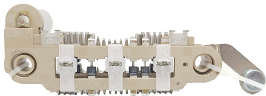
FA-MI-1413 Placa Mitsubishi A860T19370 Mitsubishi Mirage Diesel- Peugeot. CON DIODO AUXILIAR
