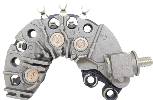
FA-V-1631 Placa Valeo 2650144, 2650236 Buick, Pontiac, Saturn CON DIODO AUXILIAR
