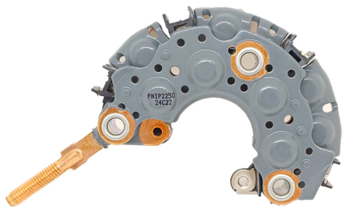
FA-N-1503 Placa Nippondenso 021580-2250. Honda Civic, Acura Toyota - Isuzu - Chevrolet - Daihatsu Suzuki. CON DIODO AUXILIAR
