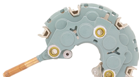
FA-N-1508 Placa Nippondenso 021580-4040-4100-4430-4690 Lexus, Toyota. CON DIODO AUXILIAR
