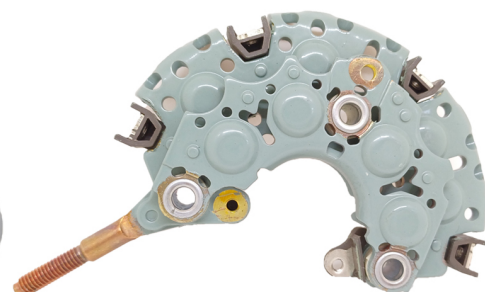
FA-N-1514 Placa Nippondenso 021580-5040 Chrysler; Dodge Jeep CON DIODO AUXILIAR
