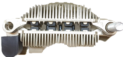
FA-MI-1429 Placa Mitsubishi A860T39970; A860T33970 Nissan, Ford Transit CON DIODO AUXILIAR
