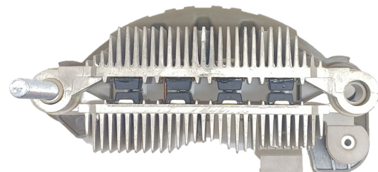
FA-MI-1443 Placa Mitsubishi A3TA4191 Chrysler; Dodge CON DIODO AUXILIAR
