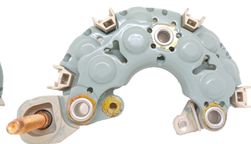
FA-N-1520 Placa Nippondenso 021580-4120. Dodge Van CON DIODO AUXILIAR
