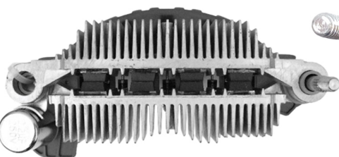
FA-MI-1467 Placa Mitsubishi A860T41370 Mitsubishi; Ford CON DIODO AUXILIAR
