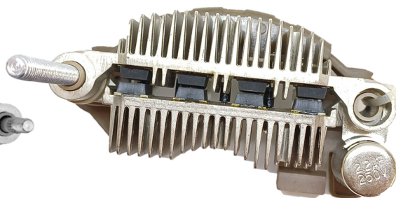
FA-MI-1468 Placa Mitsubishi A860T39270 Chrysler; Nissan; Mitsubishi CON DIODO AUXILIAR
