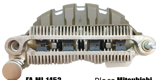
FA-MI-1453 Placa Mitsubishi A860T30170 Mitsubishi; Subaru CON DIODO AUXILIAR
