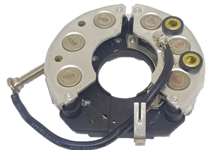
FA-B-0906 Placa Bosch 9121080595 VW CON DIODO AUXILIAR
