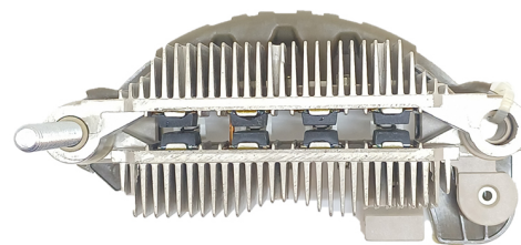
FA-MI-1412 Placa Mitsubishi A3T14292. Chrysler CON DIODO AUXILIAR
