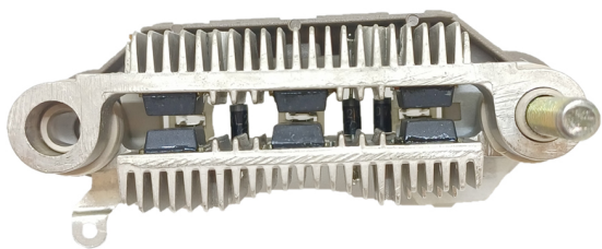
FA-MI-1446 Placa Mitsubishi A860T17170 Nissan CON DIODO AUXILIAR
