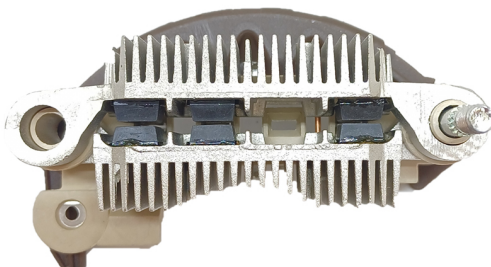
FA-MI-1486 Placa Mitsubishi A860X70970 Chevrolet, Honda, Suzuki Vitara CON DIODO AUXILIAR
