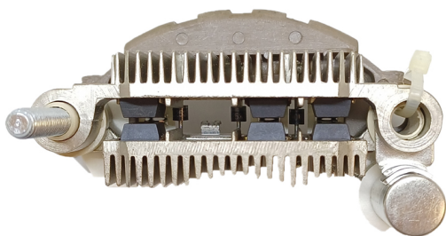
FA-MI-1425 Placa Mitsubishi A860t31570 Subaru Justy Mitsubishi Montero Diesel CON DIODO AUXILIAR
