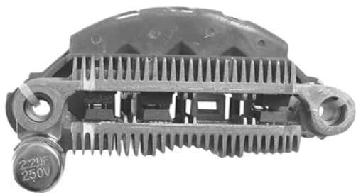
FA-MI-1422 Placa Mitsubishi A860T28670. Ford Tempo, Taurus, Sable, Transit, Mondeo, Escort. CON DIODO AUXILIAR
