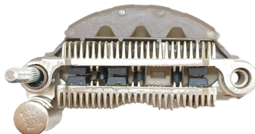
FA-MI-1481 Placa Mitsubishi A860T28770 Ford, Mazda, Dodge CON DIODO AUXILIAR
