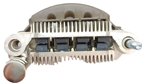
FA-MI-1457 Placa Mitsubishi A860T32570 Honda, Suzuki CON DIODO AUXILIAR
