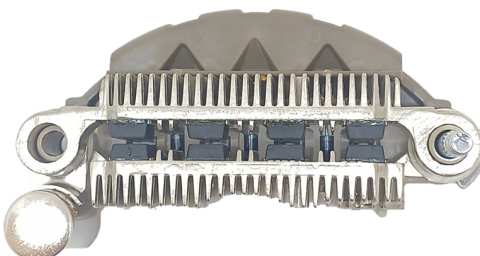
FA-MI-1441 Placa Mitsubishi A3T01691 Mazda; Subaru CON DIODO AUXILIAR
