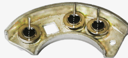
FA-100 NEGATIVA Placa tipo Argelite 28-42 amp Peugeot-Citroen Renault
