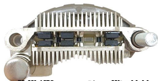
FA-MI-1470 Placa Mitsubishi A860T46570; A860X46570 Mazda; Mitsubishi CON DIODO AUXILIAR
