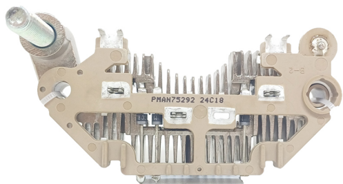
FA-MA-1353 Placa Mando Bobcat 6675292, 6678205 Bobcat, y Alternadores Mando 90A CON DIODO AUXILIAR
