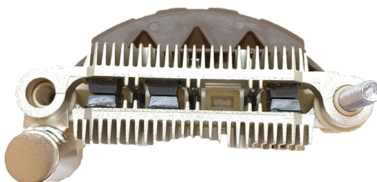
FA-MI-1450 Placa Mitsubishi A860T23170; MD611585 Mitsubishi CON DIODO AUXILIAR
