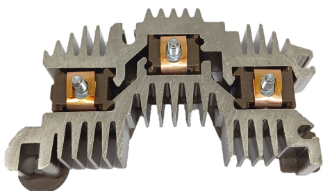
FA-DE-1107 Placa Delco 10469265, D3929 Alternadores Delco series 21SI, 22SI, 23SI 31SI, 33SI, 34SI, 35SI; IR/EF. CON DIODO AUXILIAR
