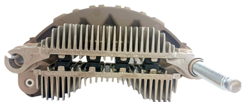
FA-MI-1479 Placa Mitsubishi A4TA8494, A4TA0594, A4TA0592 Iveco Stralis CON DIODO AUXILIAR
