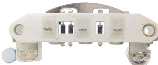
FA-MI-1435 Placa Mitsubishi A860T08770; A860T15170 Mazda; Mitsubishi CON DIODO AUXILIAR
