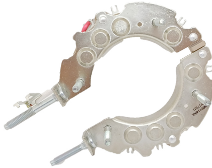
FA-N-1528 Placa Nippondenso 021590 1890, 021590 1990, 021590 1910 Toyota Hilux CON DIODO AUXILIAR
