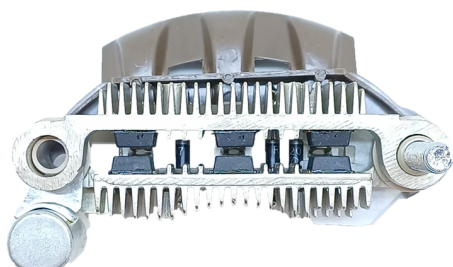
FA-MI-1485 Placa Mitsubishi A860T27170, 28370 Ford, Dodge Mitsubishi, Mazda, Hyundai, Kia CON DIODO AUXILIAR
