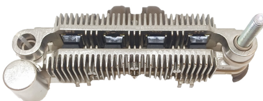
FA-MI-1420 Placa Mitsubishi A860T26070 Dodge, Hyundai. Mitsubishi. CON DIODO AUXILIAR
