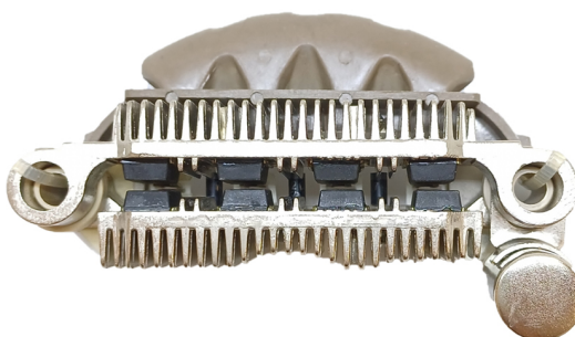
FA-MI-1456 Placa Mitsubishi A860T30870 Ford CON DIODO AUXILIAR
