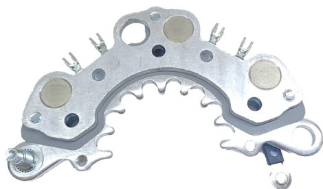
FA-H-1227 Placa Hitachi GD214675G Nissan, automotores e industriales. CON DIODO AUXILIAR
