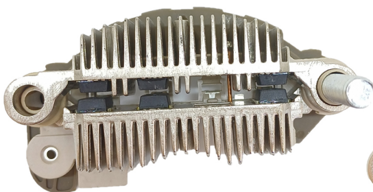
FA-MI-1471 Placa Mitsubishi A860T57870 Kia; Mazda CON DIODO AUXILIAR
