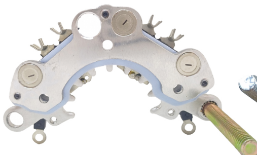
FA-H-1261 Placa Hitachi Prestolite Indiel K01208, 35214571. Corsa / VW Gol Senda Saveiro CON DIODO AUXILIAR
