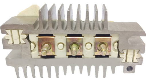
FA-DE-1128 Placa Delco 1867531 Chevrolet CON DIODO AUXILIAR
