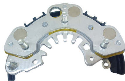
FA-H-1205 Placa Hitachi L180G-7320 Nissan Altima, Axess CON DIODO AUXILIAR
