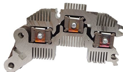
FA-DE-1103 Placa Delco 10472095 Alternadores Delco serie CS144, 124-140A IR/EF. CON DIODO AUXILIAR
