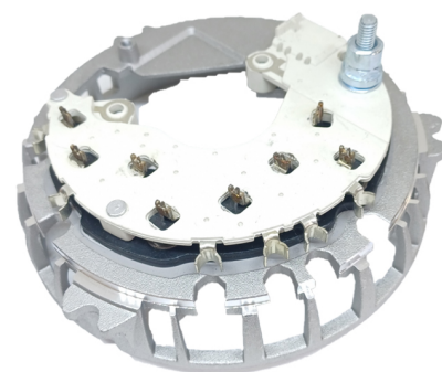
FA-F-1152 Placa Ford F8AU-10A366-AAIP Ford CON DIODO AUXILIAR
