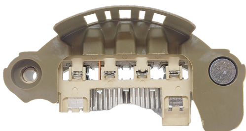
FA-MI-1482 Placa Mitsubishi A860X78370 Citroën Berlingo C4 C5 Xsara. Peugeot 206 207 301 307 407 Partner CON DIODO AUXILIAR
