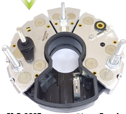
FA-B-0925 Placa Bosch 1127320590; 1127320977. Scania CON DIODO AUXILIAR
