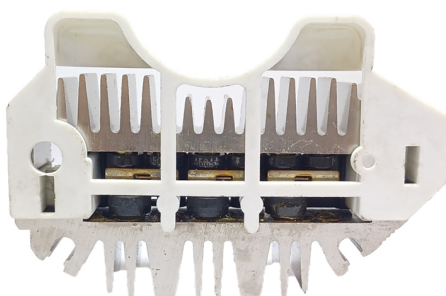
FA-DE-1129 Placa Delco 1985801 GM CON DIODO AUXILIAR
