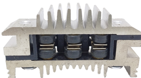
FA-V-1608 Placa Valeo 581025 /071 /078, 593074, 606625, 611197 /199 /788, 618093 /439 /503 /720, 690260 /971. NC013, NC014, CON DIODO AUXILIAR
