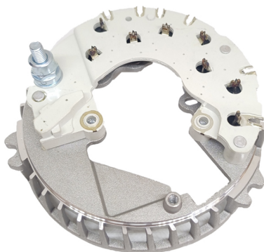
FA-F-1151 Placa Ford F8WU-10A366-AAIP. Ford CON DIODO AUXILIAR
