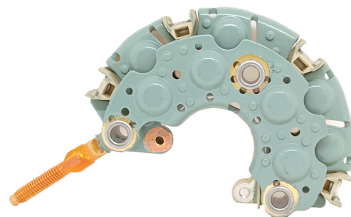
FA-N-1502 Placa Nippondenso 021580-2160; 021580-2230 Acura, Honda, Isuzu, Toyota, Sterling CON DIODO AUXILIAR
