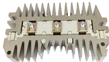
FA-DE-1112 Placa Delco 801816 Alternadores Delco serie 27SI, tipos 100, 200; y series 29SI, 30SI Negativo a masa. IR/EF. CON DIODO AUXILIAR
