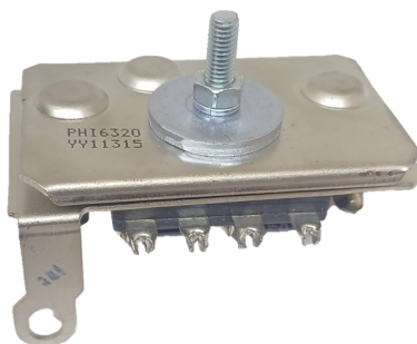
FA-H-1249 Placa Hitachi L140N-13201,-13202. Nissan. CON DIODO AUXILIAR
