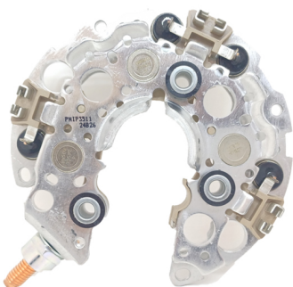
FA-N-1524 Placa Nippondenso RTF40172 Ford, Mazda, Volvo CON DIODO AUXILIAR
