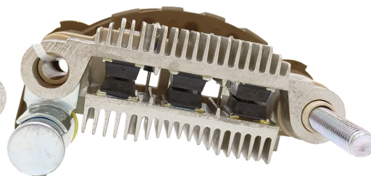
FA-MI-1418 Placa Mitsubishi A860T22770 Subaru CON DIODO AUXILIAR
