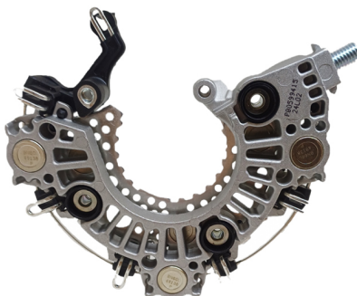
FA-B-1001 Placa Bosch F00M573933 M Benz BMW Mini Cooper CON DIODO AUXILIAR
