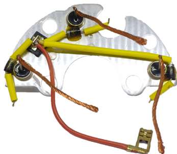
FA-B-0988 Placa Bosch 9121450587 Volkswagen Gol Passat, Voyage CON DIODO AUXILIAR
