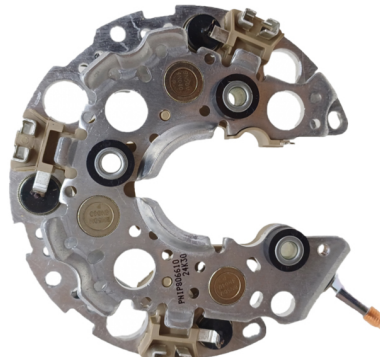
FA-N-1534 Placa Nippondenso 021580-6610 Toyota Camry, Corolla, Rav 4 CON DIODO AUXILIAR
