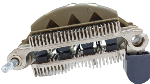
FA-MI-1423 Placa Mitsubishi A860T29970, A860X29999, A860X35099 Nissan. CON DIODO AUXILIAR
