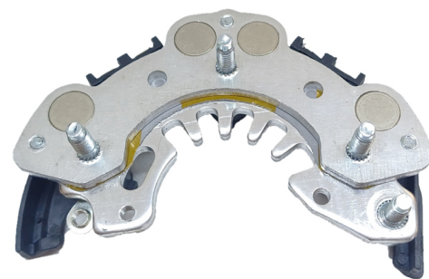
FA-H-1226 Placa Hitachi L170-33202 Subaru CON DIODO AUXILIAR
