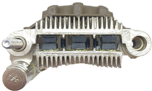
FA-MI-1410 Placa Mitsubishi A860T11970, A860T13370 Ford, mazda, mitsubishi. CON DIODO AUXILIAR
