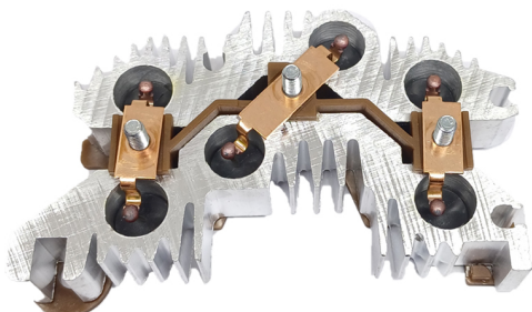
FA-DE-1110 Placa Delco 10470609, D3992 trabajo pesado Alternadores Delco serie 21SI, 22SI, 23SI, CS144 IR/EF CON DIODO AUXILIAR
