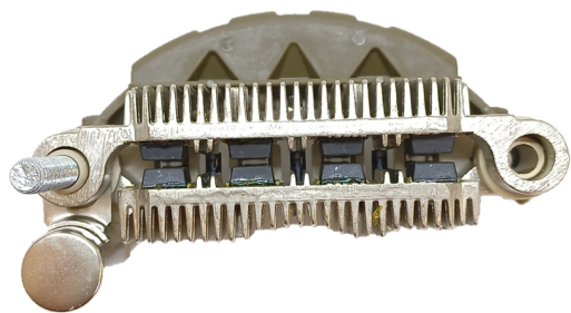
FA-MI-1458 Placa Mitsubishi A2T32962 Ford; Peugeot CON DIODO AUXILIAR
