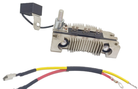
FA-MM-1305 Placa Marelli 63022101, 63622101 Peugeot Renault CON DIODO AUXILIAR
