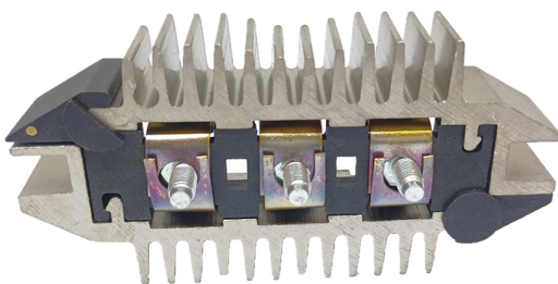
FA-DE-1126 Placa Delco 3493008 Opel CON DIODO AUXILIAR
