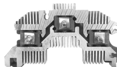
FA-DE-1109 Placa Delco 10470609, D3992 Alternadores Delco serie 21SI, 22SI, 23SI CS144 IR/EF. CON DIODO AUXILIAR
