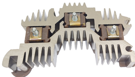
FA-DE-1123 Placa Delco 1988976, D3987 Camiones Ford; Mack; Volvo; Caterpillar CON DIODO AUXILIAR
