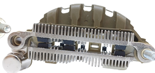
FA-MI-1463 Placa Mitsubishi A860T36070 Mitsubishi CON DIODO AUXILIAR
