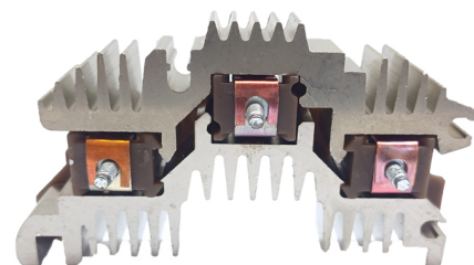
FA-DE-1124 Placa Delco 10471170 Chevrolet Blazer Camiones; Hummer CON DIODO AUXILIAR
