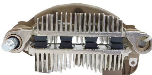
FA-MI-1477 Placa Mitsubishi A860X45170 Infiniti, Nissan CON DIODO AUXILIAR
