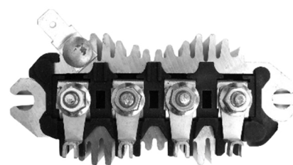
FA-V-1627 Placa Valeo A105612A, A105947A Renault, Porsche CON DIODO AUXILIAR
