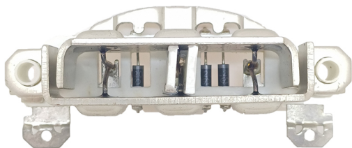
FA-MI-1434 Placa Mitsubishi A860T08470 Nissan CON DIODO AUXILIAR
