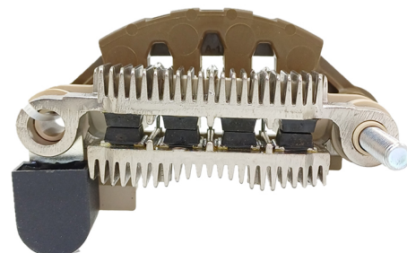
FA-MI-1421 Placa Mitsubishi A860T27270 Nissan Pulsar. CON DIODO AUXILIAR
