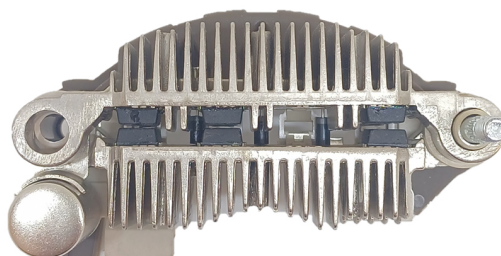
FA-MA-1351 Placa Mando AB170066, AB180092 Kia CON DIODO AUXILIAR
