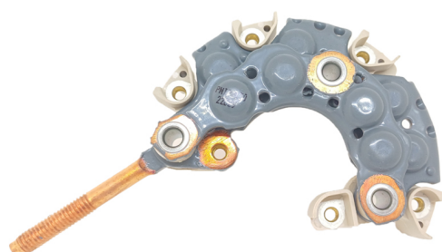
FA-N-1505 Placa Nippondenso 021580-3130 Daihatsu, Acura Toyota - Isuzu - Honda CON DIODO AUXILIAR
