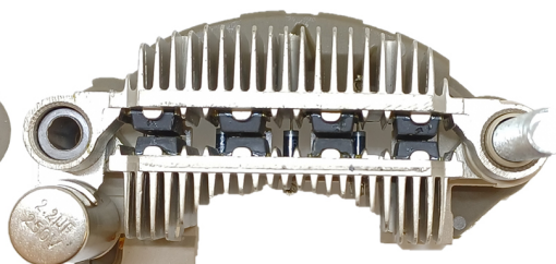
FA-MI-1466 Placa Mitsubishi A860T39070, A860X44170, MD618811 Ford; Mazda; Mitsubishi CON DIODO AUXILIAR
