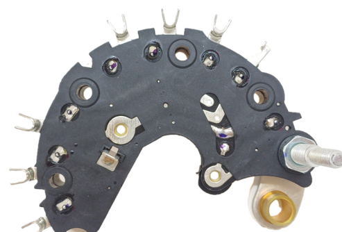
FA-V-1621 Placa Valeo 545937, 592847, 2545938 Peugeot; Renault CON DIODO AUXILIAR
