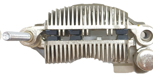
FA-MI-1475 Placa Mitsubishi A002T81391 Chrysler; Mitsubishi CON DIODO AUXILIAR
