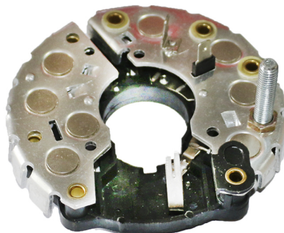
FA-B-0908 Placa Bosch 1127320700.Fiat Ford 1632835 Audi CON DIODO AUXILIAR
