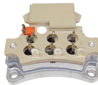
FA-F-1155 Placa Ford E43Z10304A; E6DZ10304A. Ford Pick Up CON DIODO AUXILIAR
