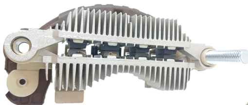
FA-MI-1408 Placa Mitsubishi A3T-N1791 Ford Transit CON DIODO AUXILIAR
