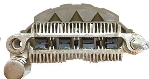
FA-MI-1451 Placa Mitsubishi A860T23270; MD611586 Mitsubishi; Hyundai; Dodge CON DIODO AUXILIAR
