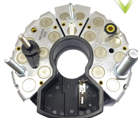
FA-B-0939 Placa Bosch 1127320920; 1127320954. Cummins, John Deere. CON DIODO AUXILIAR
