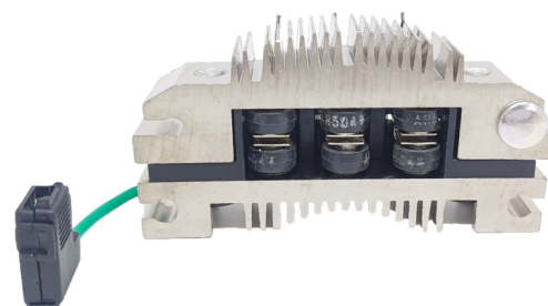
FA-MM-1304 Placa Marelli 63622001 Fiat CON DIODO AUXILIAR
