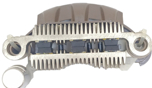
FA-MI-1449 Placa Mitsubishi A860T17770, 17770 Ford; Chrysler Mitsubishi CON DIODO AUXILIAR
