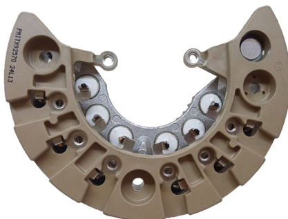
FA-MI-1489 Placa Mitsubishi A860X92570. Ford Fiesta CON DIODO AUXILIAR
