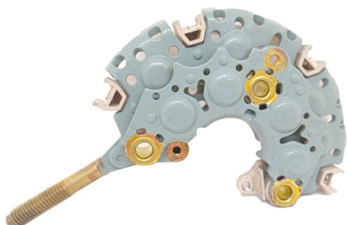
FA-N-1512 Placa Nippondenso 021580-4610, 5040 Toyota Hilux, Land Cruiser CON DIODO AUXILIAR
