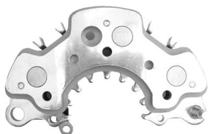
FA-H-1233 Placa Hitachi L1100G-23201; LR1100-711B Nissan CON DIODO AUXILIAR
