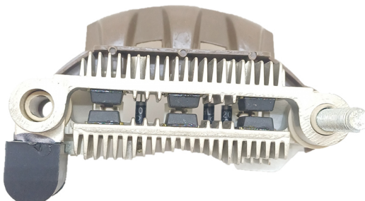
FA-MI-1444 Placa Mitsubishi A860T13470, 16470 Nissan CON DIODO AUXILIAR
