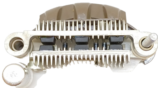
FA-MI-1452 Placa Mitsubishi A860T24570 Mitsubishi; Dodge CON DIODO AUXILIAR
