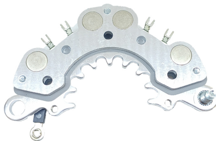
FA-H-1207 Placa Hitachi L190G-33204 Nissan 240 Sx CON DIODO AUXILIAR
