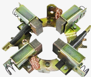
PCB-123 PORTA ESCOBILLAS ARRANQUE T. BOSCH, M-BENZ Mod. NUEVO 24v 10 x 22 x 19 (9 001 083 596)
