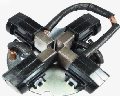
PCB-33 C/Carb. Indiel Motor Maxion Ford M93R Peugeot 504 505 DF-100 Ranger JSX-31-32 Fijacion : 46
