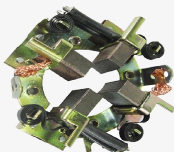
PCB-02 S/Carb. PCB-02-1 C/Carb. M. Benz Arranque JF Cod. 9001083392 BSX-433 Fijacion : 58
