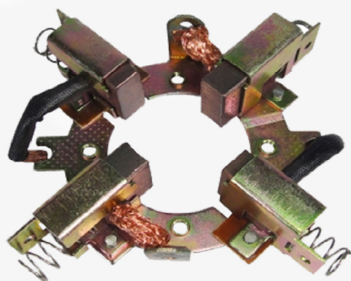
PCB-21 S/Carb. PCB-21/1 C/Carb. M/Benz Bosch Fiat Volvo Iveco VW BSX-592 Ford Cargo Camiones Orig 9001083569 Fijacion : 58
