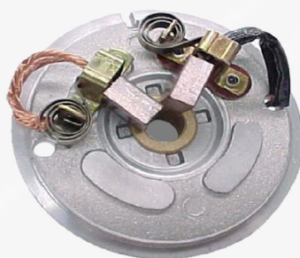
PCB-16 S/Carb. PCB-16/1 C/Carb. Renault Cerrada Arranque Garef USX-21-22
