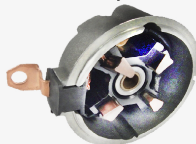
PCB-20 C/Carb. Arranque Bosch Wapsa VW Gol Ford Escort Orig 246012 X-213-2 Fijacion : 45
