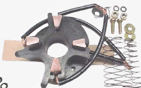
PCB-05 S/Carb. PCB-05-1 C/Carb. Frontal Indiel Ford Sierra R11 VW Renault 11 Chico LASX-40-41 Fijacion : 43 Bakelita
