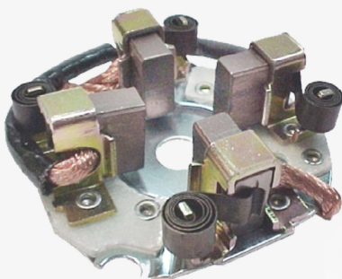
PCB-39 C/Carb. M. Marelli Ducato Tipo Uno Citroen Berlingo JSX-31-32 Fijacion : 46 (020)
