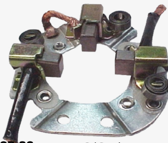
PCB-38 C/Carb. Marelli Fiat Palio Siena Uno Nafta JSX-35-36 Orig83224461 Fijacion : 45 (34.34)
