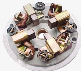
PCB-26 C/Carb. Arranque Wapsa Volkswagen Senda Saveiro Gol Diesel Carb. 213/5
