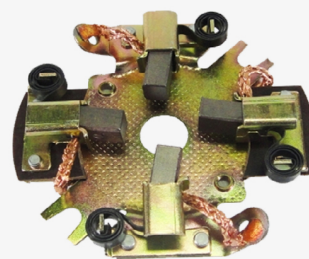
PCB-03 C/Carb. Fiat 147 Duna Uno Ford Escort GM VW Gold Senda Cód. 9001082239 BSX-75 Fijacion : 46
