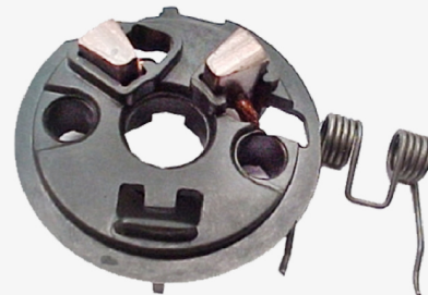
PCB-14 s/Carb PCB-14/1 c/Carb. Renault 19 D Arranque Valeo Frontal Peugeot D6RA PSX-148-149 Fijacion :38
