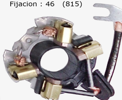
PCB-47 C/Carb.(C/G P/G) Bosch Fiat Duna Uno Ford Escort Clio D Expres Scenic DW1.7KW BSX-157-158 Fijacion : 43 (956)
