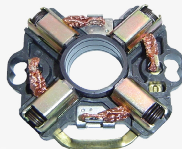
PCB-49/1 C/Carb. Bosch Motor Maxion camiones IVECO BSX-165 9003334341 Fijacion : 48 (918)
