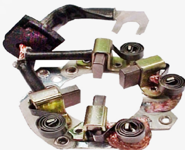
PCB-19/1 C/Carb. Arr. Indiel Hitachi R-19 Duna Clio Corsa Peugeot 205-306 405 Boxer Fiat 147 Palio Siena Orig. 35258566 HISX 8128 Fijacion :56
