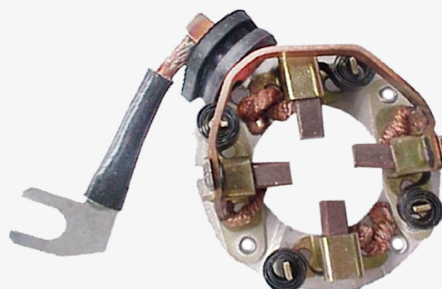
PCB-41 C/Carb. Motorcraf Ford Ka Fiesta Escort Transit FX -341. Fijacion : 52 (341)
