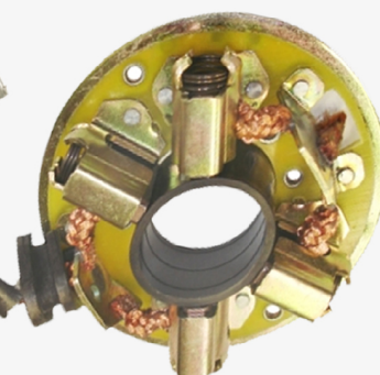
PCB-58 C/Carb. BOSCH Iveco Daily Ford F250 MWM ORIG6033AD0368 (162)
