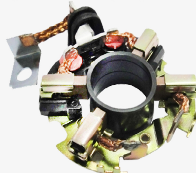
PCB-44 C/Carb. (C/C P/G) Bosch Ford Escort Polo Gol Saveiro Corsa Berlingo Peugeot 205 306 405 Partner BSX-161-162 Der 9001081094 Fijacion : 46 (815)
