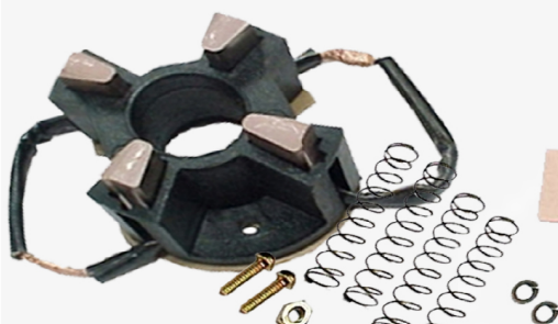
PCB-04 S/Carb. PCB-04-1 C/Carb. Frontal Indiel G Ford Taunus F-100 Torino Fiat LASX-43-44 Fijacion : 47 Bakelita
