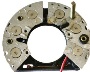
FA-860 VW Gol - Ford Escort. Alternador 55 Amp. Reemp. 3682
