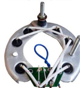
FA-700 Peugeot-Renault- Ford Reg.Inc. Alternador 70 A.
