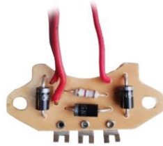
FA-310 Placa auxiliar 55-90 amp uso gral 35213293
