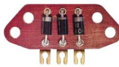
FA-310 Placa auxiliar 55-90 amp uso gral 35213293
